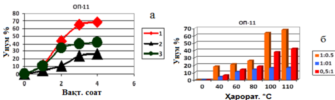
2-расм. Кислород сақлаган органик модификаторнинг чиқиш унумига эпихлоргидрин ва натрий карбонатнинг нисбатлари 1) 1:0,5; 2) 1:0,1; 3) 0,5:1 бўлганда вақтнинг ва хароратнинг таъсири.
