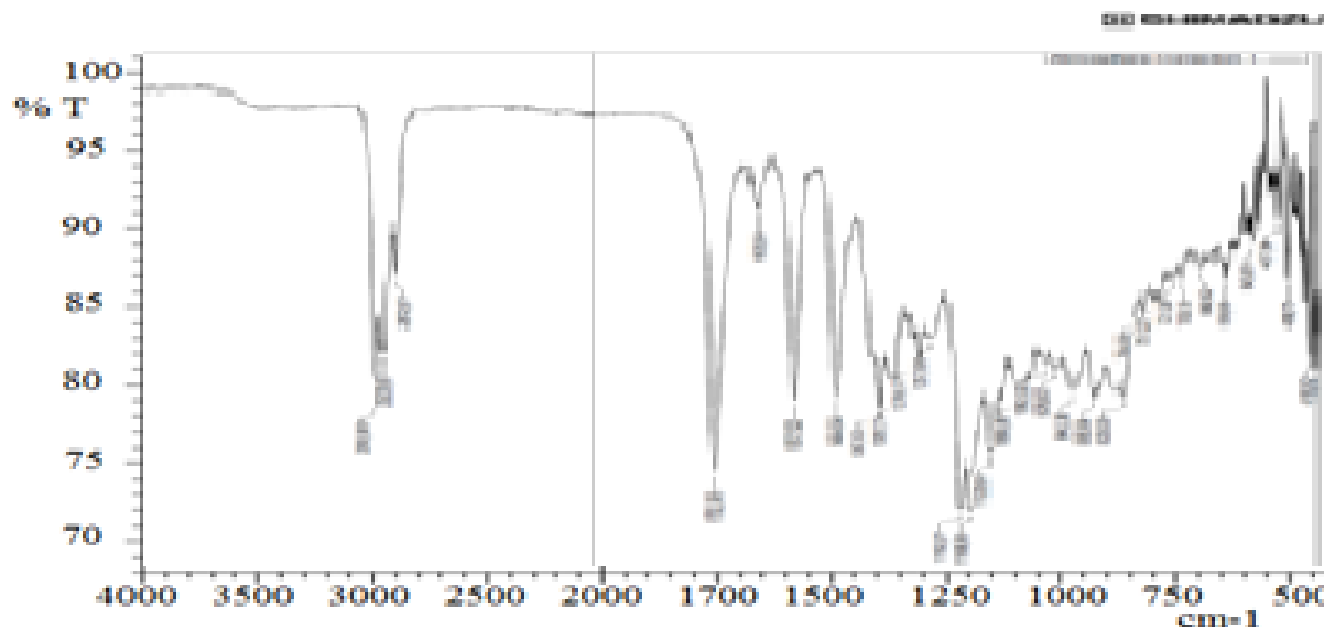
3-расм. Азот сақлаган органик модификаторнинг ИҚ спектри, УНДж-20.
