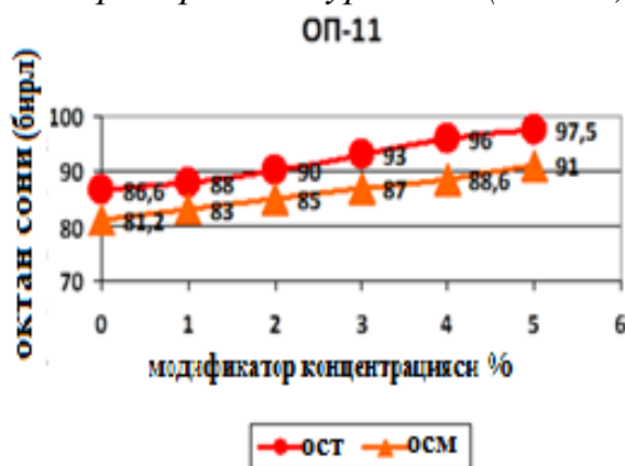
5-расм. ОП-11 қўшилганда реформат октан сонини ўзгариши.
