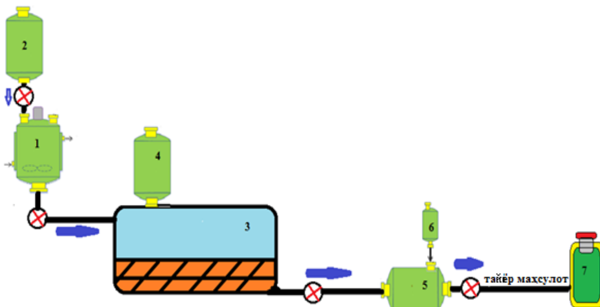
8-расм. ОП-12 маркали кислород сақлаган модификатор олиш технологик схемаси.
