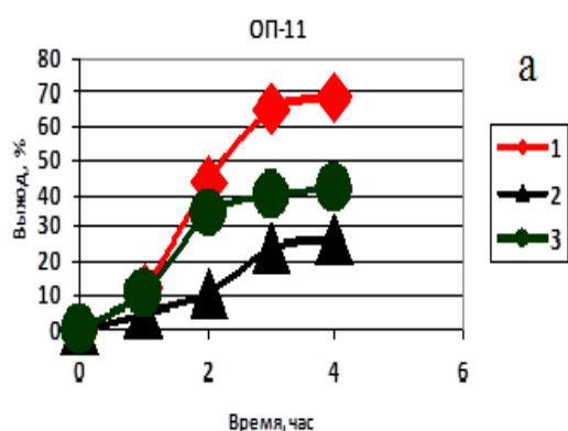
Рисунок 2. Зависимость выхода кислородсодержащего органического модификатора от времени и температуры при соотношении эпихлоргидрин : карбонат натрия: 1) 1:0,5; 2) 1:0,1; 3) 0,5:1.
