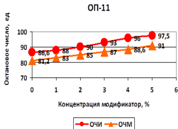
Рисунок. 5. Изменение октанового числа реформата при добавке ОП-11.
