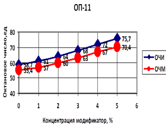
Рис. 4. Изменение октанового числа прямогонной бензиновой фракции при добавке ОП-11.
