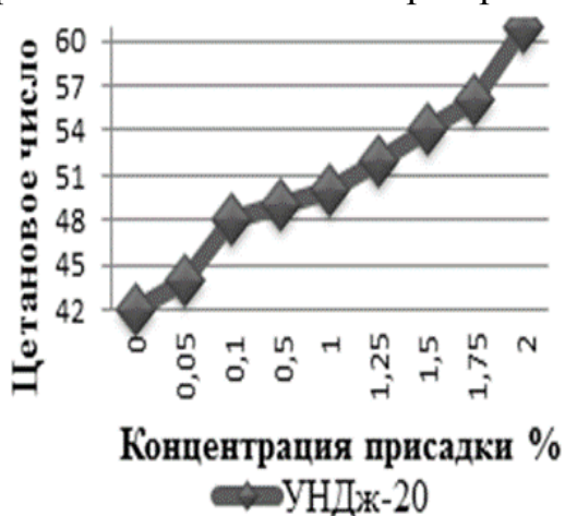
Рисунок 6. Изменение цетанового числа в присутствии УНДж-20.
