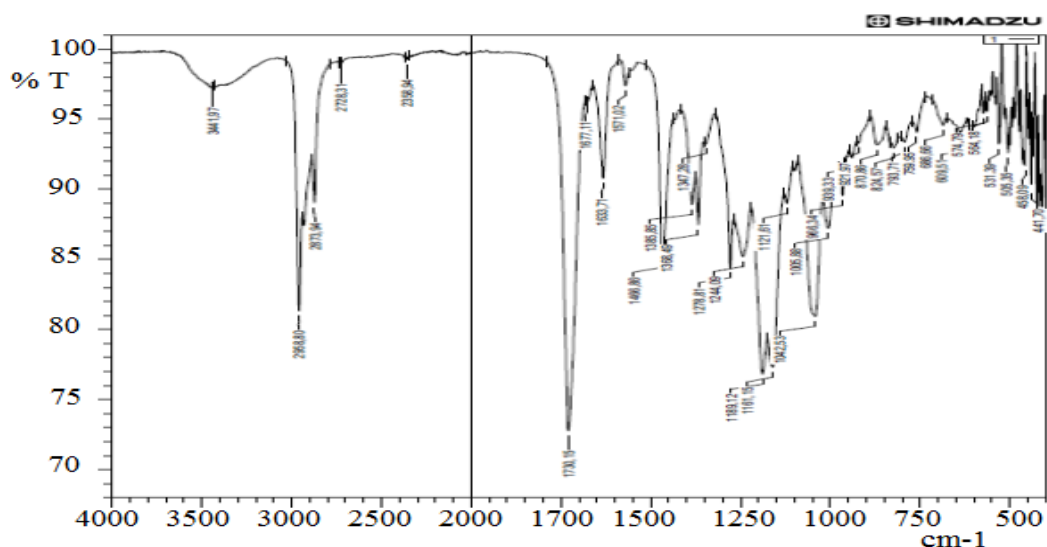
1-расм. ОП – 10 маркали кислород сақлаган органик модификаторнинг ИҚ – спектри.
