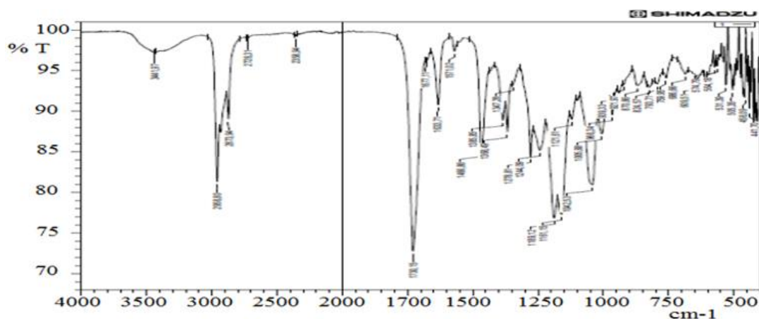
Рисунок 1. ИК-спектр кислородсодержащего органического модификатора марки ОП–10.
