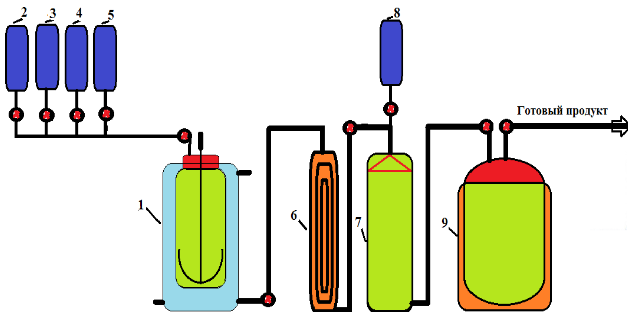
Рисунок 9. Технологическая схема получения цетаноповышающего и антикоррозионного модификатор марки УНДж-20.
