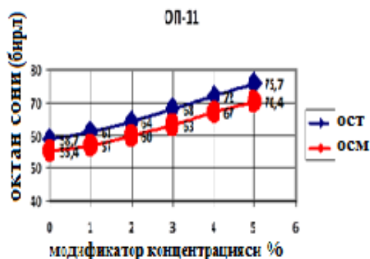
4-расм. ОП-11 қўшилганда тўғридан-тўғри хайдалган бензин фракциясининг октан сонини ўзгариши.
