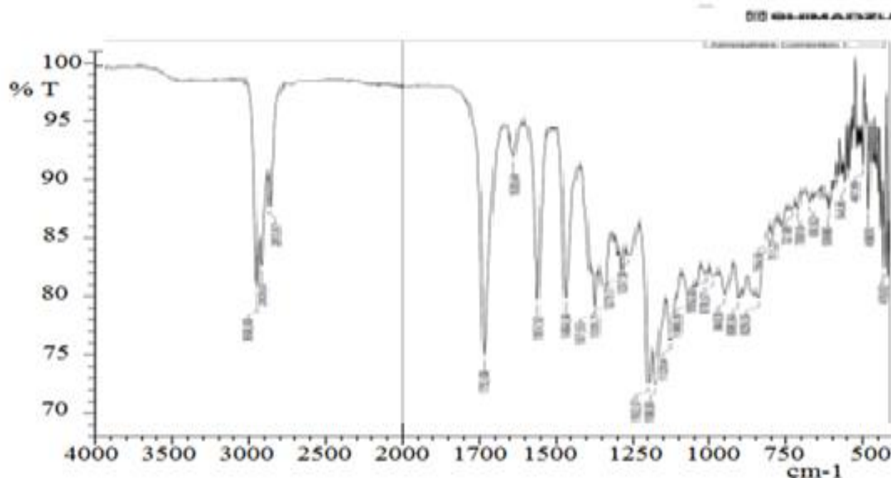
Рисунок 3. ИК-спектр азотсодержащего органического модификатора, УНДЖ-20.
