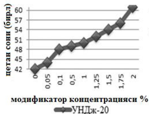
6-расм. УНДж-20 ёрдамида дизел ёқилғисининг цетан сони ўзгариши.
