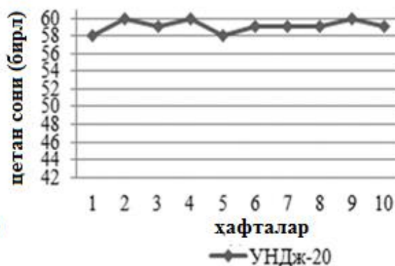
7-расм. Цетан сонини оширувчи модификаторларни сақлашдаги барқарорлиги.
