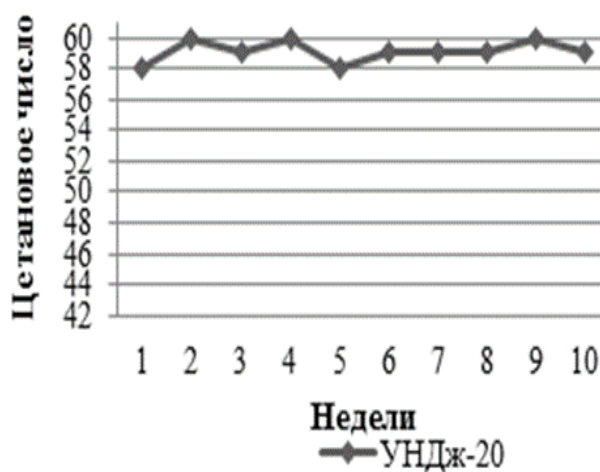
Рисунок 7. Стабильность при хранении цетаноповышающих присадок.
