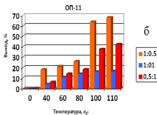
Рисунок 2. Зависимость выхода кислородсодержащего органического модификатора от времени и температуры при соотношении эпихлоргидрин : карбонат натрия: 1) 1:0,5; 2) 1:0,1; 3) 0,5:1.
