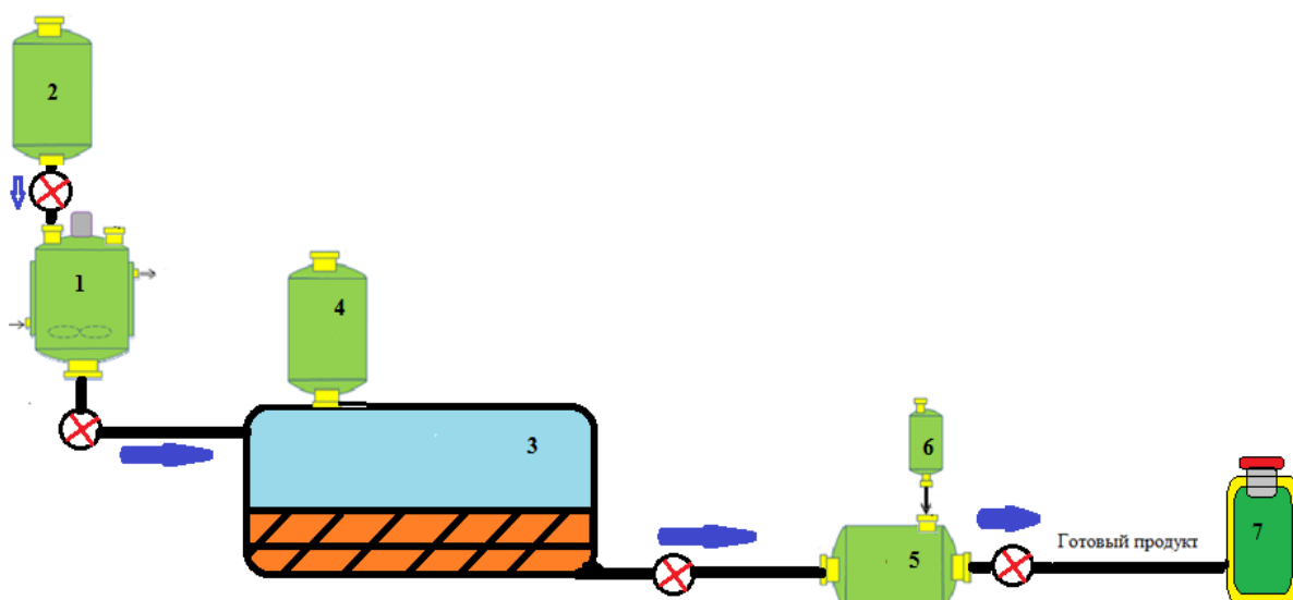
Рисунок 8. Технологическая схема получения кислородсодержащего модификатора марки ОП-12.
