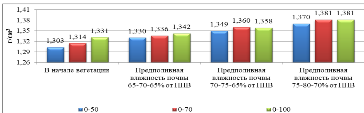
Рисунок 2. Объемная масса почвы в начале и конце вегетации при возделывании повторной культуры сои, г/см 3 (2017-2019 гг).
