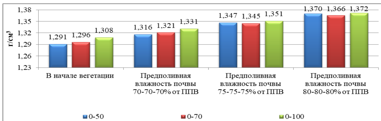
Рисунок 1. Объемная масса почвы в начале и конце вегетации при возделывании озимой пшеницы, г/см 3 (2017-2020 гг).
