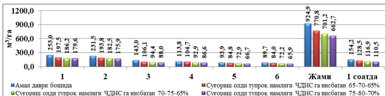
4-расм. Соя тажриба даласи тупроғининг сув ўтказувчанлиги, м 3 /га (2017-2019 йй).
