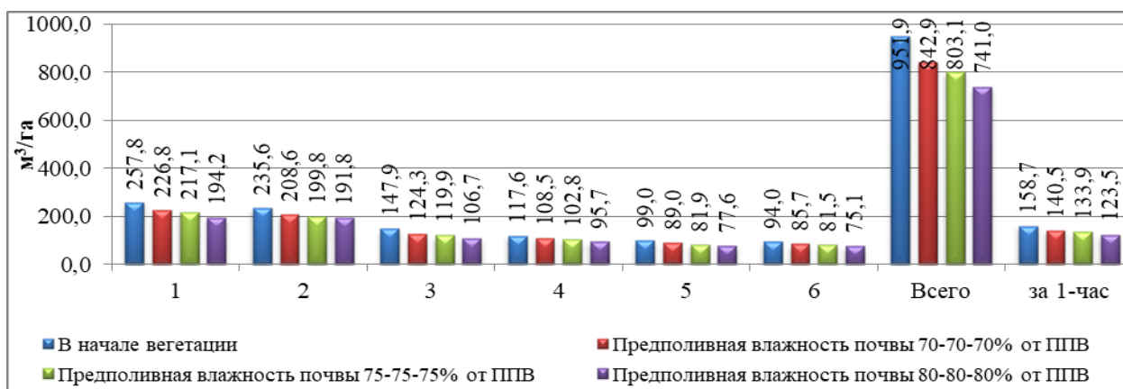
Рисунок 3. Водопроницаемость почвы опытного участка озимой пшеницы, м 3 /га (2017-2020 гг).
