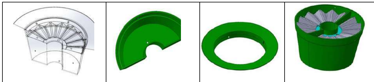
Рис. 4. Модифицированная полезная модель «Водосборное устройство». (автор М.И.Рузметов, 2021 г.)
