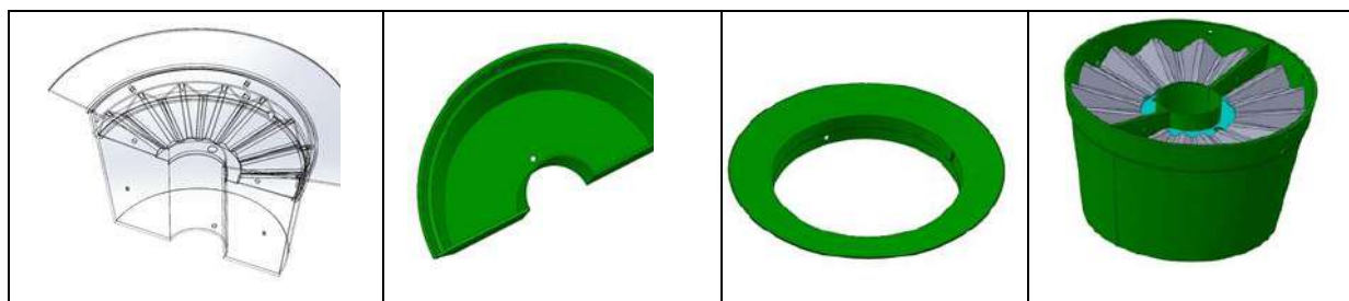
4-расм. Модификациялашган «Сув йиғиш қурилмаси» фойдали модели (муаллиф М.Рузметов, 2021 й.)
