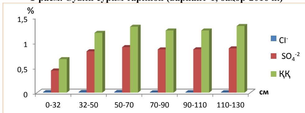
2-расм. Сувли сўрим таркиби (вариант-1, куз-2016 й.)
