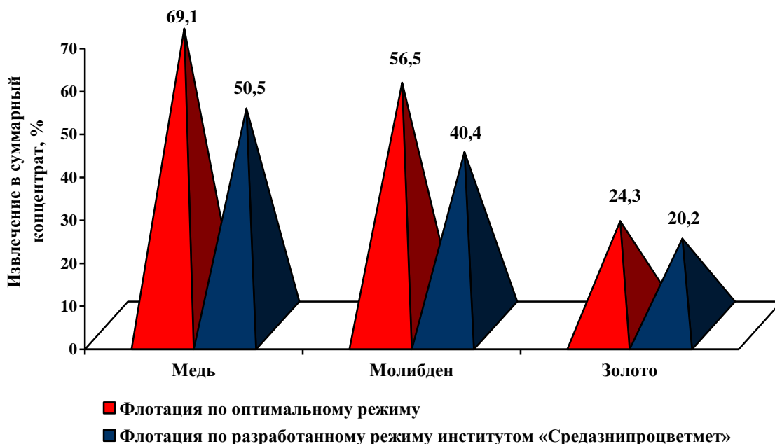
Рис. 4. Результаты флотации лежалых хвостов с двумя перечистками в замкнутом цикле
