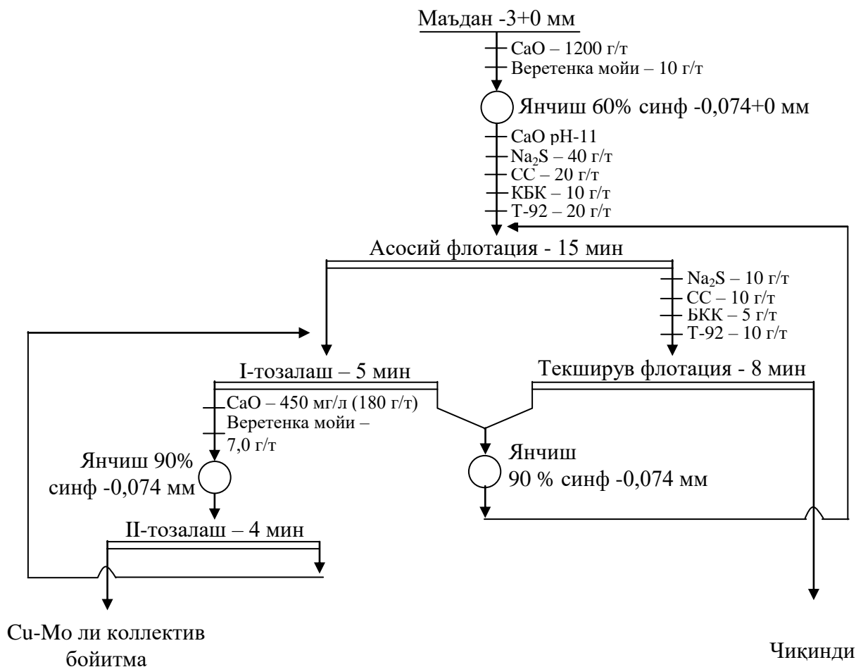
2-расм. Ёпиқ циклда Қалмоққир кони маъданини флотациялаш тажрибалари схемаси
