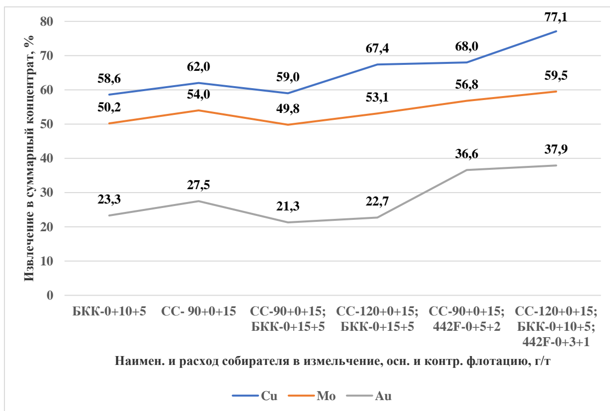
Рис. 3. Извлечение Cu, Mo и Au в суммарный пенный продукт при сравнительных опытах флотации проб лежалых хвостов с традиционными реагентами-собираелями БКК, 442F и новым реагентом СС
