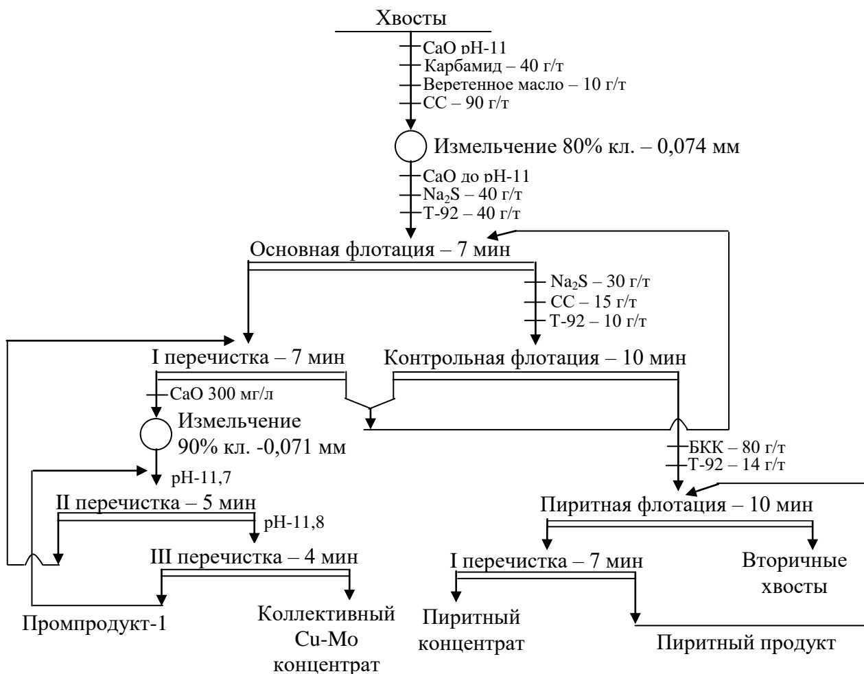
Рис. 5. Схема флотации лежалых хвостов с подавлением пирита и добавлением в качестве реагента-собирателя СС без применения БКК и 442F в стадии обогащения меди и молибдена
