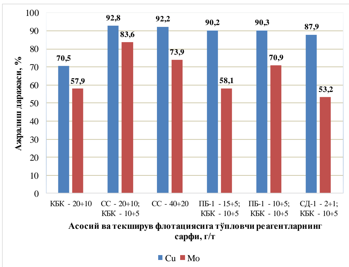
1-расм. КБК ва янги СС, ПБ-1, СД-1 реагентлари билан мис-молибден маъдани намунасини флотациялашнинг солиштириш тажрибаларида асосий флотация бойитмасига Cu ва Mo ни ажралиши
