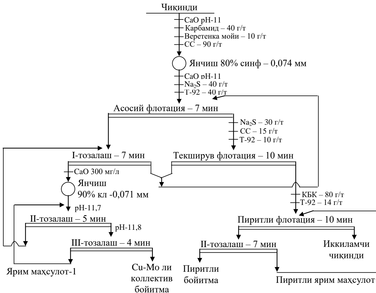
5-расм. Мисни ва молибденни бойитиш циклида пиритни сўндириш билан ва КБК ва 442F ни қўллагасдан тўпловчи реагент сифатида СС ни қўшиб чиқиндиларни флотациялаш схемаси
