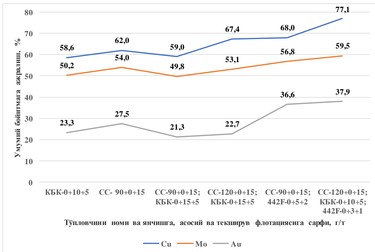
3-расм. Анъанавий тўпловчи реагентлар КБК, 442F ва янги СС реагенти билан чиқиндилар намуналарини флотациялаш бўйича солиштириш тажрибаларида Cu, Mo и Au умумий кўпикли маҳсулотга ажралиши
