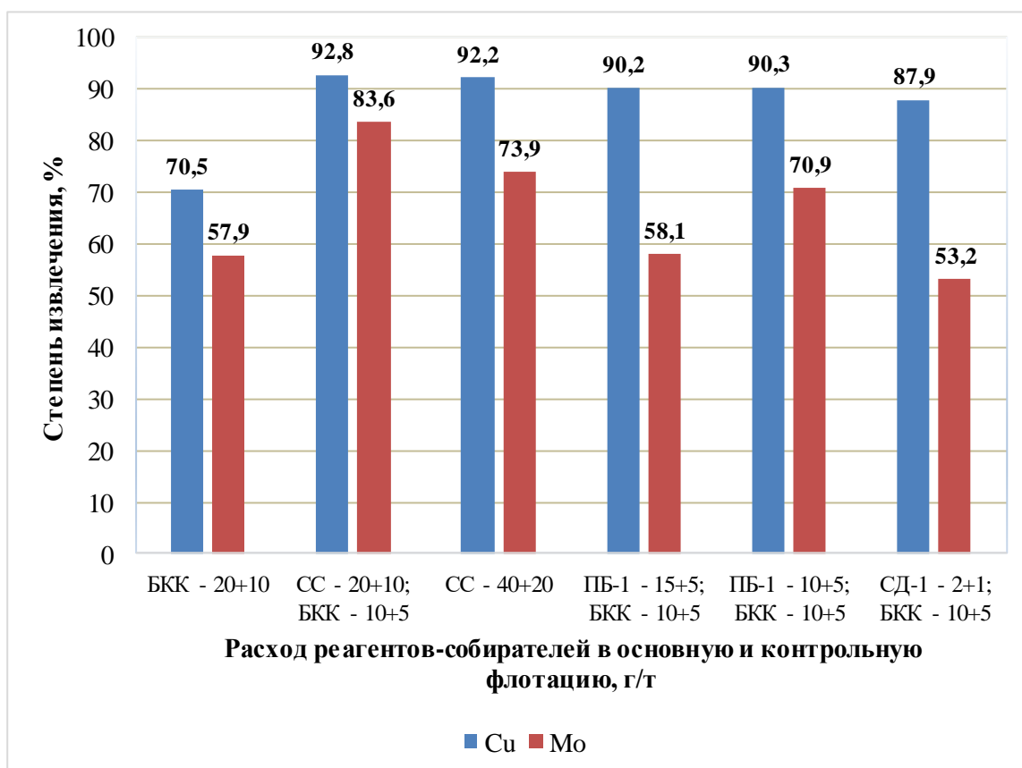
Рис. 1. Извлечение Cu и Mo в концентрат основной флотации при сравнительных опытах флотации проб медно-молибденовой руды с БКК и новыми реагентами СС, ПБ-1 и СД-1
