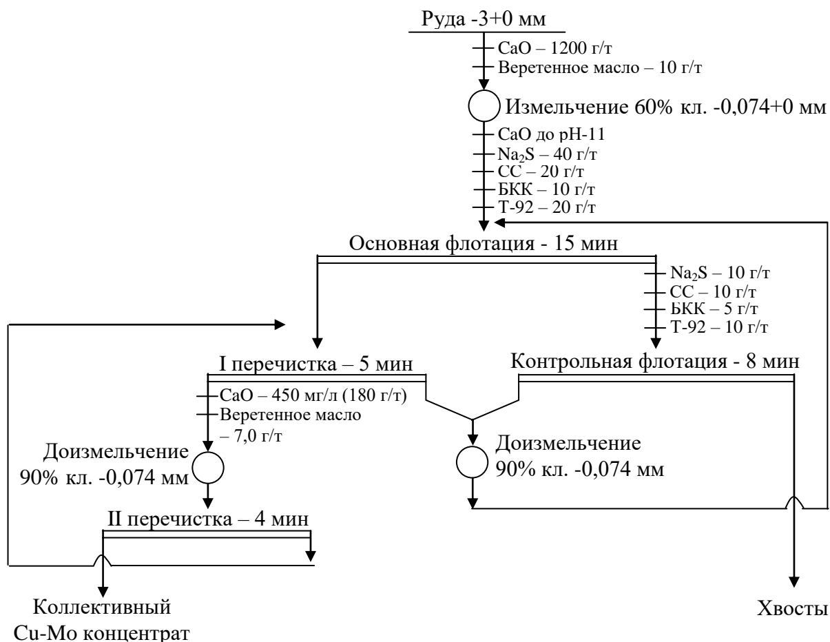
Рис. 2. Схема опытов флотации руды месторождения Кальмакыр в замкнутом цикле
