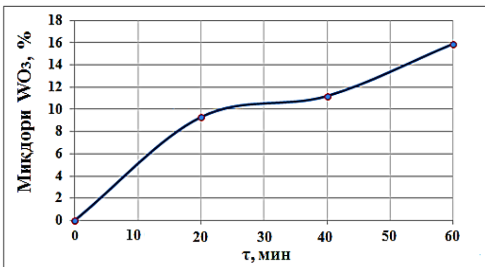
3-расм. Ўтказилган тажрибаларда кекдан вольфрам ажратиб олишнинг жараёнлар давомийлигига боғлиқлиги (винтли сепараторда)
