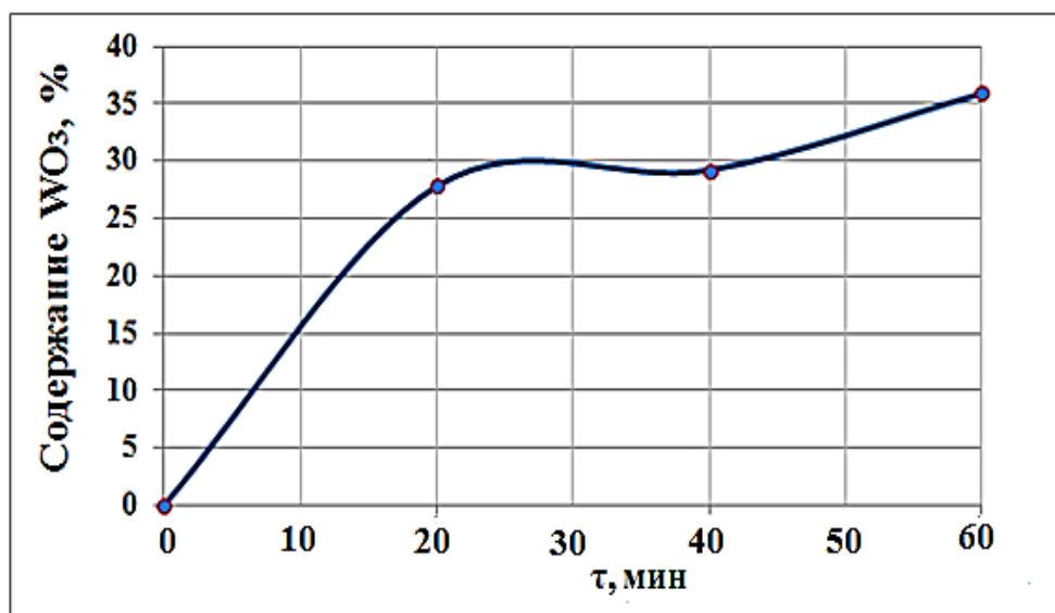
Рис. 2. Зависимость извлечения вольфрама из лежалых хвостов от продолжительности процесса (3 опыта последовательно)
