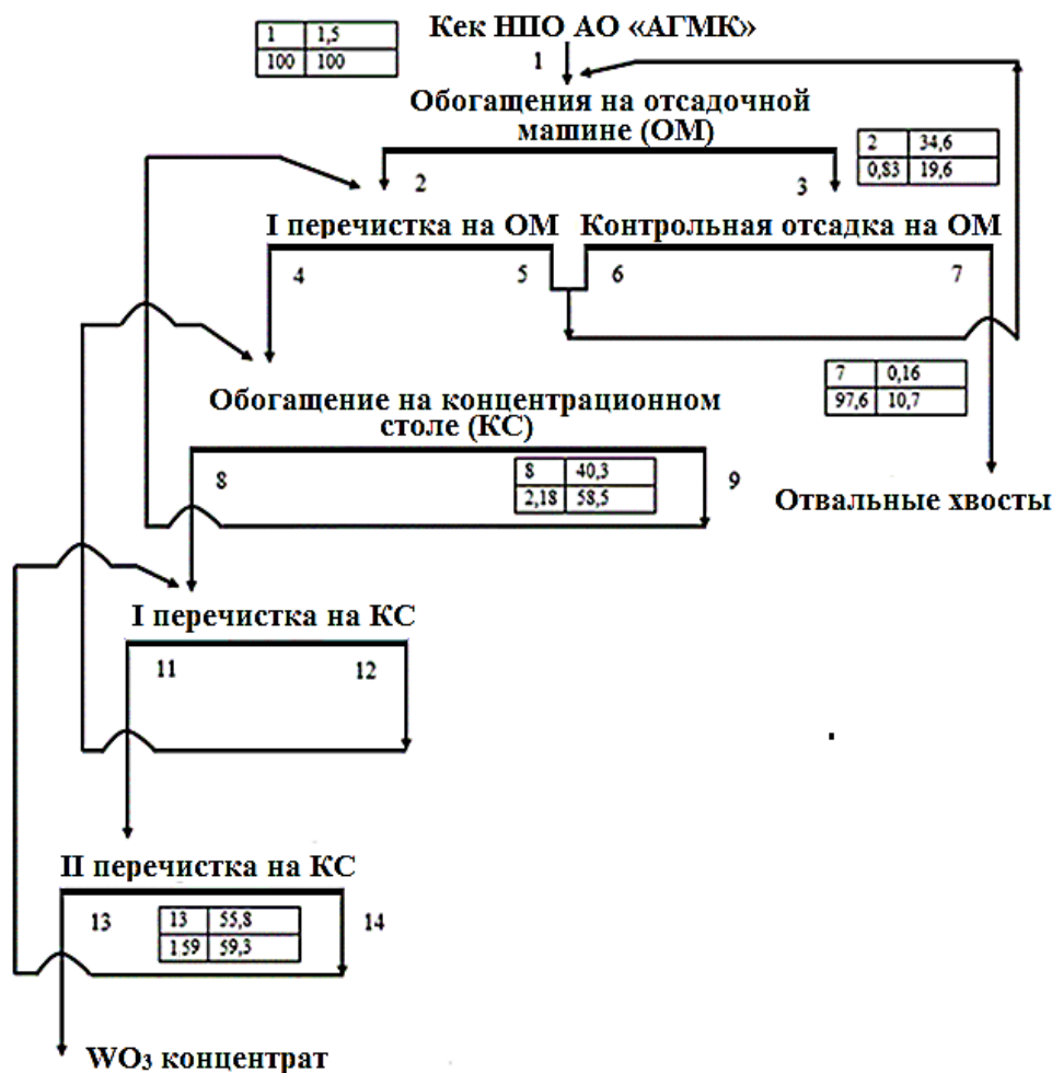
Рис. 11. Качественно-количественная схема и материальный баланс рекомендуемой технологической схемы обогащения кека НПО АО «Алмалыкский горно-металлургический комбинат» гравитационным методом с применением отсадочной машины
