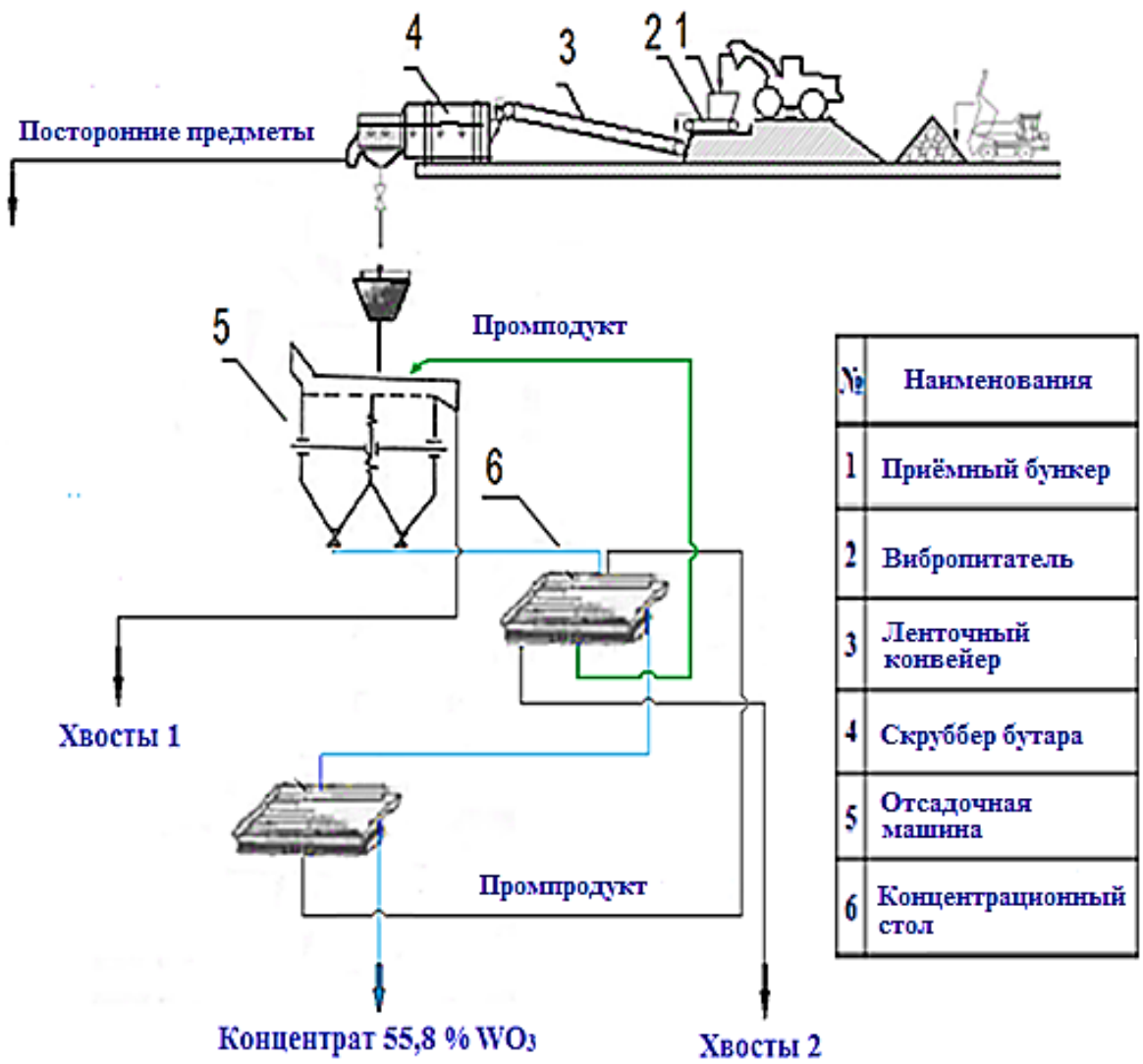
Рис. 7. Схема цепи аппаратов для укрупненно-лабораторных испытаний
