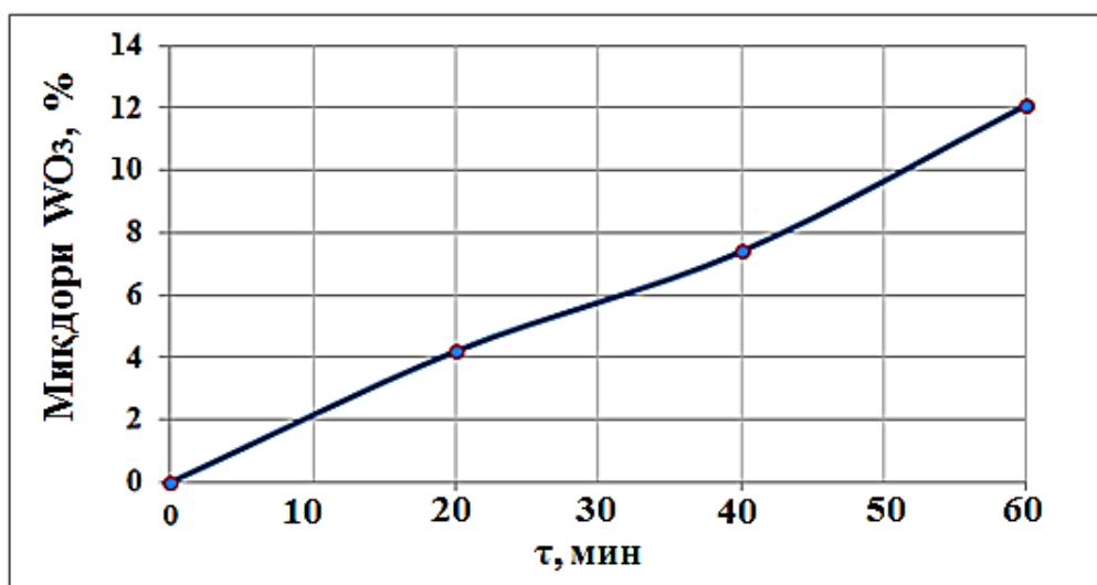
1-расм. Винтли сепараторда кўп йиллик чиқиндилардан вольфрам ажратиб олишнинг тозалашлар сони ва жараёнларнинг давомийлигига боғлиқлиги
