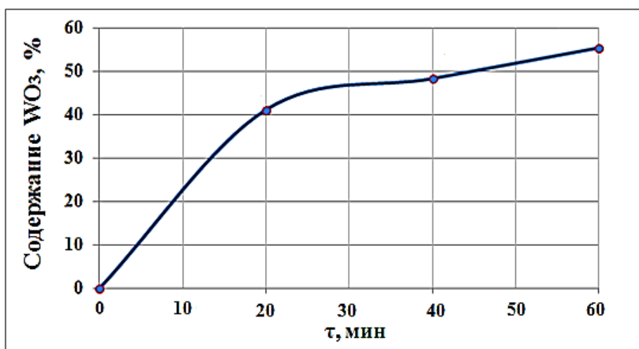
Рис. 4. Зависимость извлечения вольфрама из кеков от времени процесса в отсадочной машине
