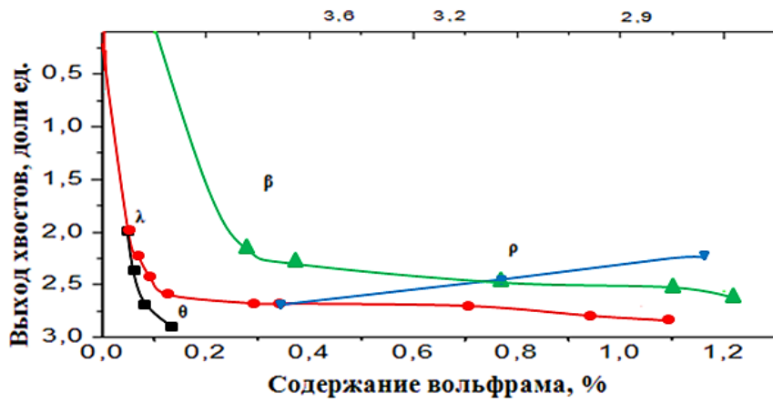
Рис. 6. Зависимость увеличения выхода кеков НПО гравитационного обогащения от содержания WO_3 для класса -1 +0,5 мм
