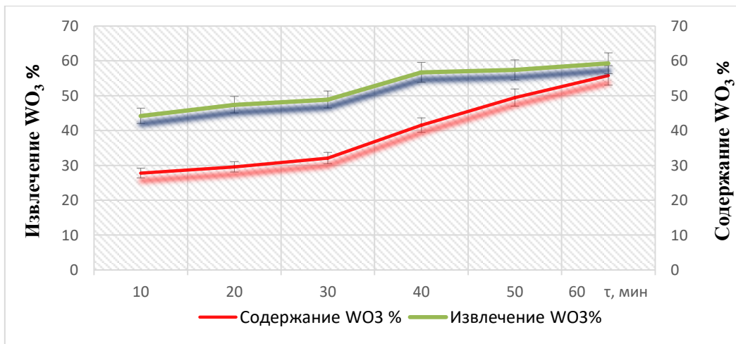
Рис. 9. Зависимость извлечения вольфрама из кека НПО на отсадочной машине от содержания WO 3 в проведенных опытах
