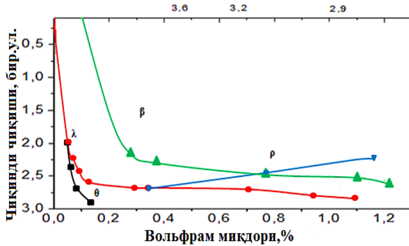
6-расм. -1+0,5 синфлар учун WO 3 миқдоридан гравитацион бойитиш кеклари чиқиншининг ошишига боғлиқлиги
