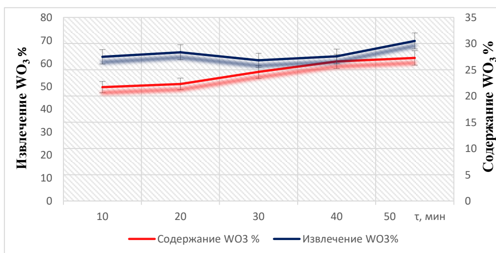
Рис. 8. Зависимость извлечения вольфрама из лежалых хвостов Ингичкинской обогатительной фабрики на отсадочной машине
