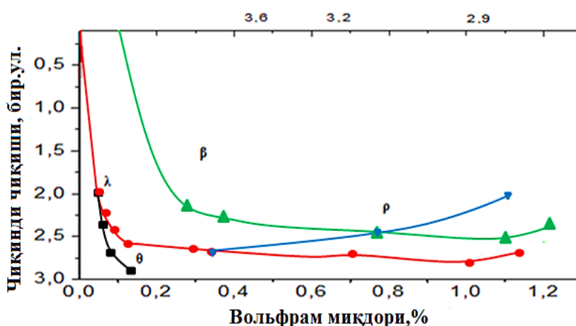
5- расм. -3+0,044 синфлар учун WO 3 миқдоридан гравитацион бойитиш чиқиндилари чиқишининг ошишига боғлиқлиги
