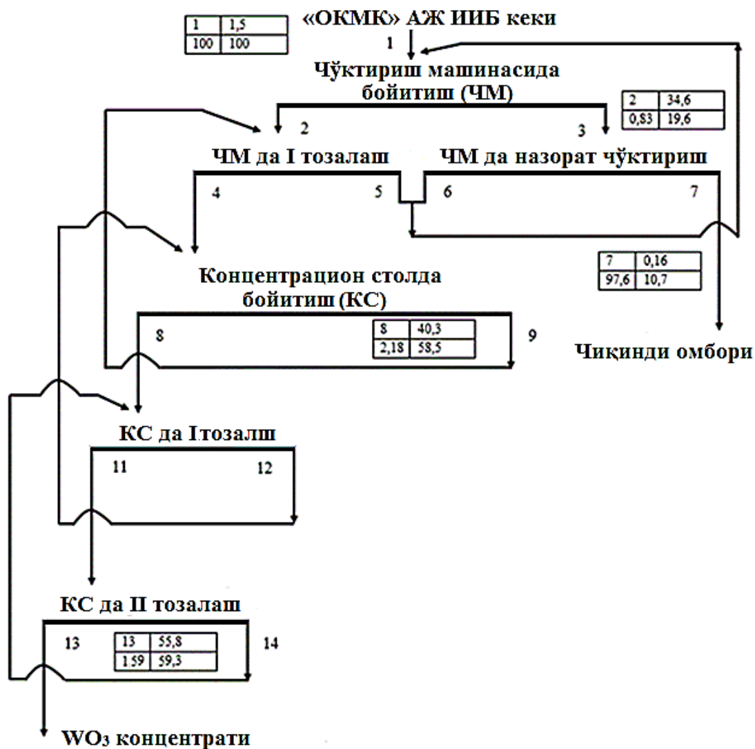
11-расм. Чўктириш машинаси билан гравитацион усулда «Олмалик кон-металлургия комбинати» АЖ ИИБ кекларни бойитиш учун тавсия этилган технологик схеманинг моддий баланси ва сифат миқдор схемаси
