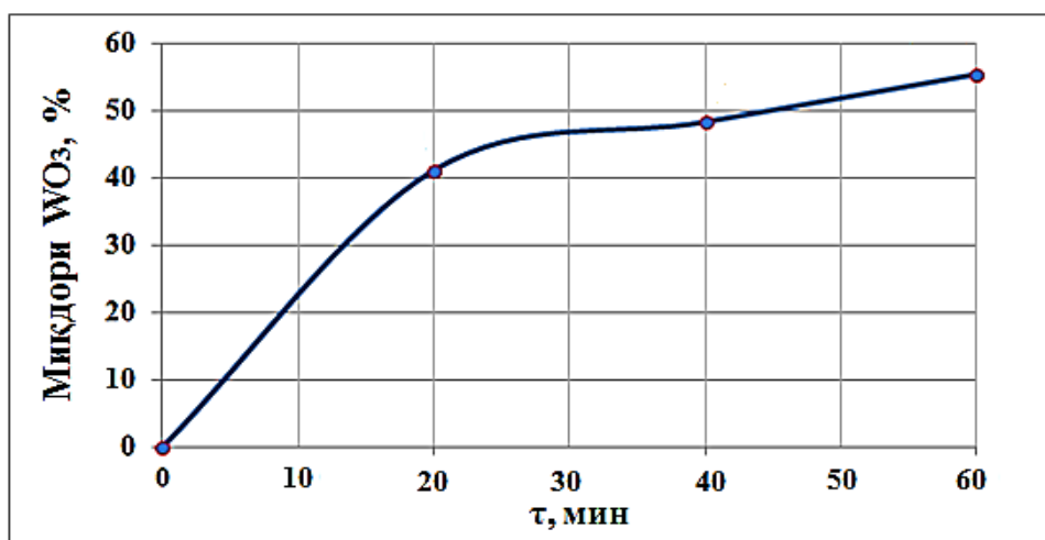
4-расм. Чўктириш машинасида кекдан вольфрам ажратиб олишнинг жараён вақтларига боғлиқлиги
