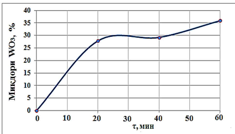
2-расм. Кўп йиллик чиқиндилардан вольфрамни ажратиб олишнинг вақт давомийлигига боғлиқлиги (3 тажриба кетма-кетлигида)
