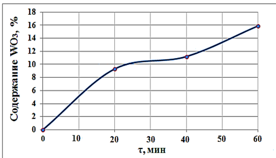
Рис. 3. Зависимость извлечения вольфрама из кеков от продолжительности процесса в проведенных опытах (на вихревом сепараторе)
