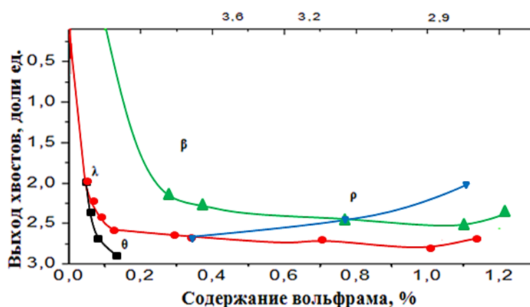
Рис. 5. Зависимость увеличения выхода хвостов гравитационного обогащения от содержания WO_3 для класса -3+0,044 мм
