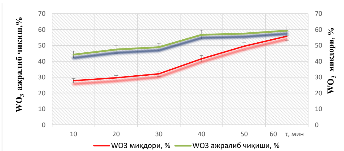
9-расм. Чўктириш машинасида ИИБ кекларидан вольфрам ажралиб чиқишининг ўтказилган тажрибалардаги WO 3 миқдорига боғлиқлиги
