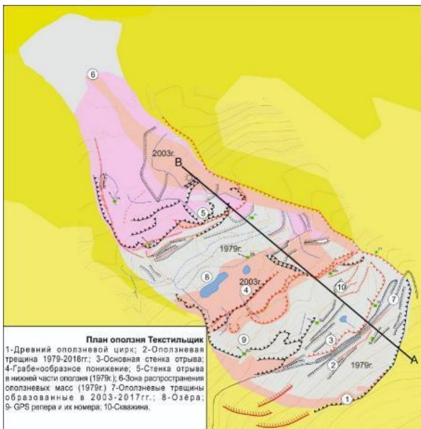
1-расм. Текстильщик кўчкиси чизмаси.
