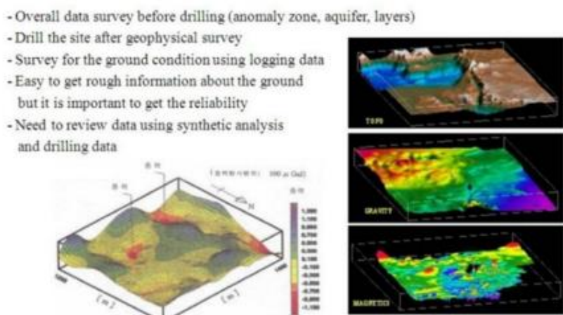
Рис. 11. Компьютерное 3D-моделирование состояния параметров оползневой массы.
