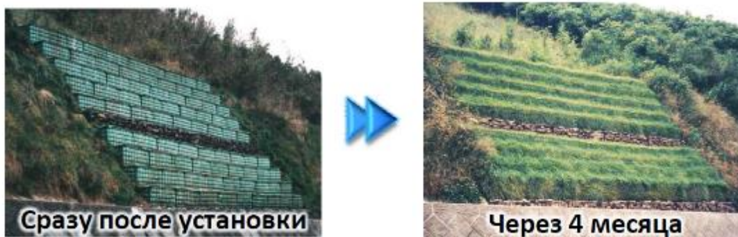
Рис. 13. Габионовая (сотовая) подпорная стенка.
