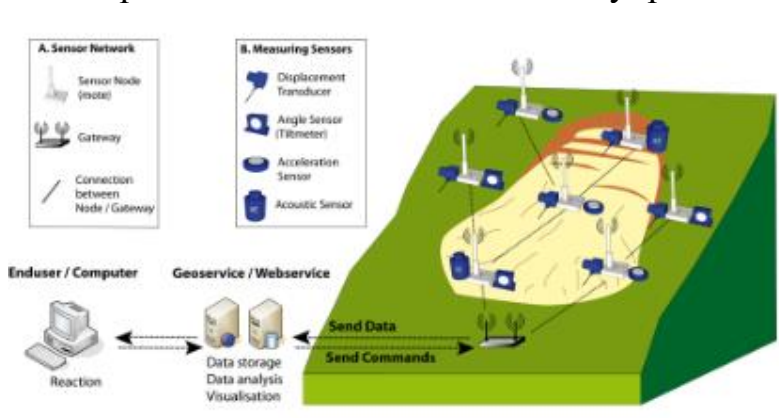
Рис. 10. Методика применения дистанционных сенсоров.
