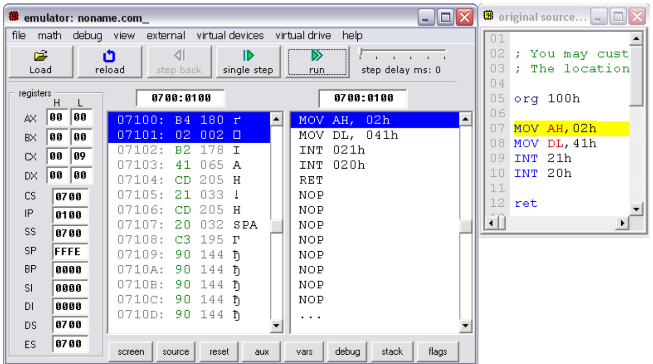
Рис. 1.2. Окно эмулятора Emu8086.
